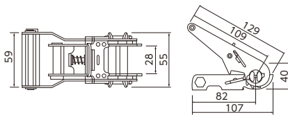
LBR100W 破断強度 1,000kgf
