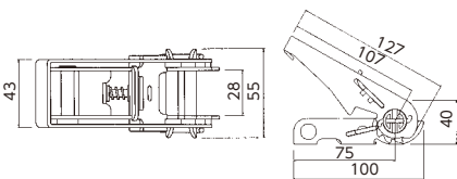
LBR100W 破断強度 1,000kgf
