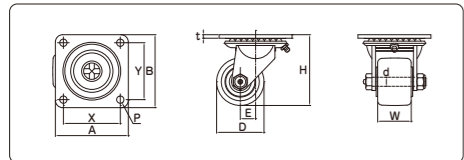
寸法図(自在車) (単位:mm)
